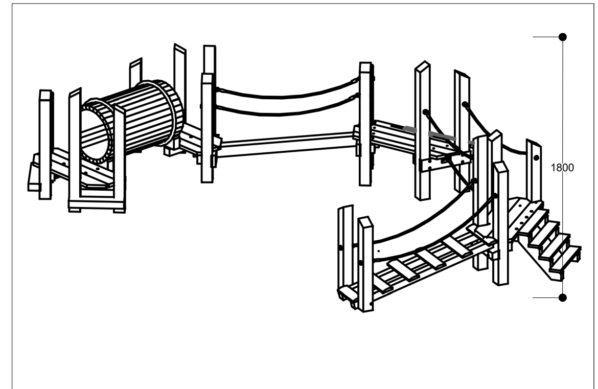
TP10 - Totter Trail - Iso 01 NTS
