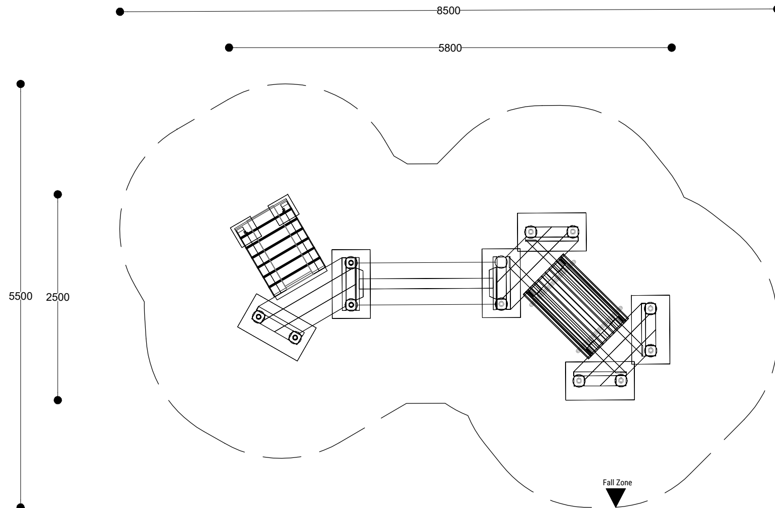
TP10 - Totter Trail - Plan 01 @1:50
