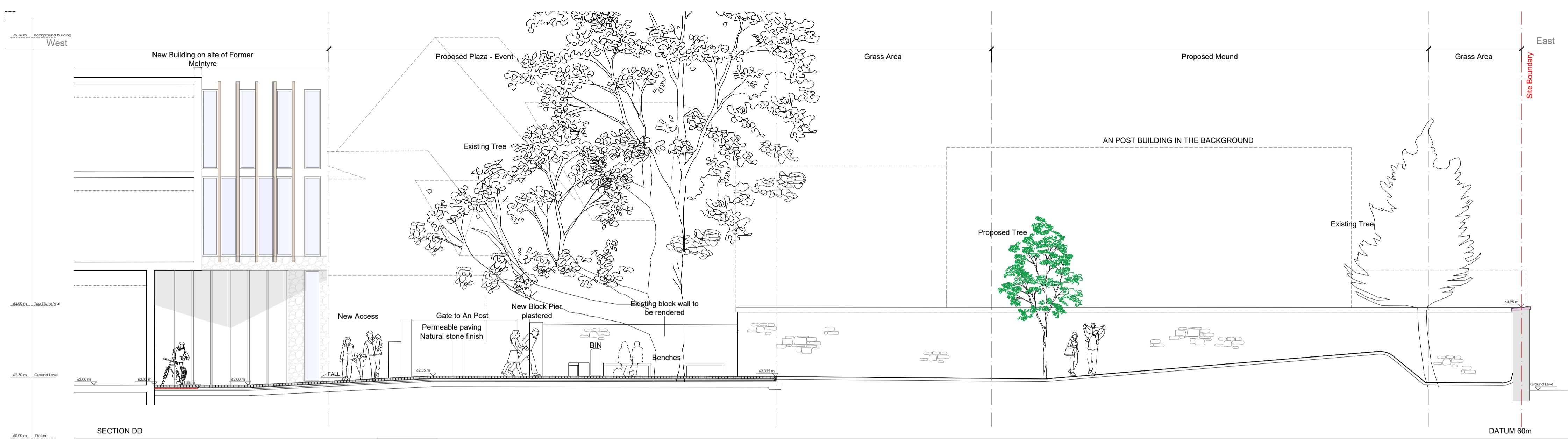
DD Proposed Section DD 242 1:100
